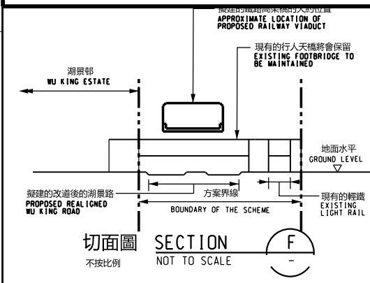
切面圖 SECTION 不按比例 NOT TO SCALE
