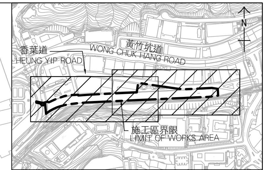
位置圖 LOCATION PLAN 比例 SCALE A1 1 : 6000
