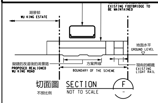
切面圖 SECTION
