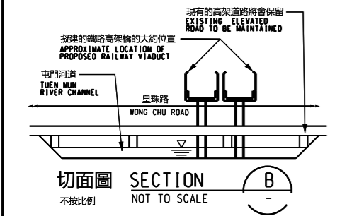
切面圖 SECTION B 不接比例 NOT TO SCALE
